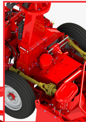
Alta tecnologia em caixas de transmissão com forte sistema de cardan
