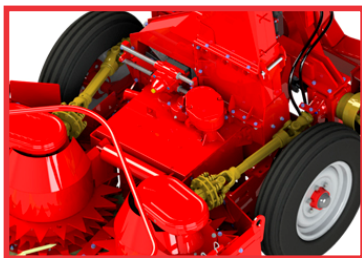
Duas rodas de apoio e eixo com pistões hidráulicos para levante da máquina
