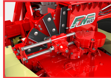
Sistema de afiação de facas que numa operação uniforme, simples e segura, afia todo o conjunto rapidamente;
