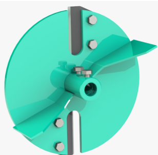
Rotor eficiente equipado con 2 cuchillas y 2 lanzadores;
