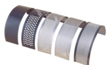
Peneiras 0.8 - 3.0 - 5.0 - 10.0 mm e fundo liso
